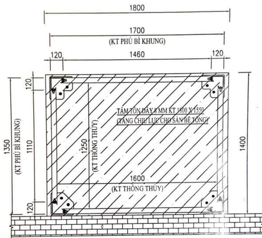
🏠 MẶT BẰNG PIT COS 00
