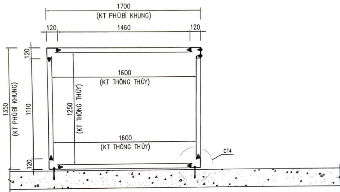
MẶT BẰNG KHUNG THÉP T2-T3-T4
