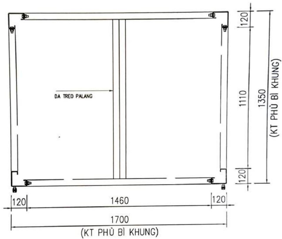
🏠 MẶT BỀ MẶT KHUNG THÉP
