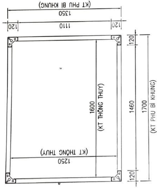
⇨ MẶT BẰNG KHUNG THÉP
